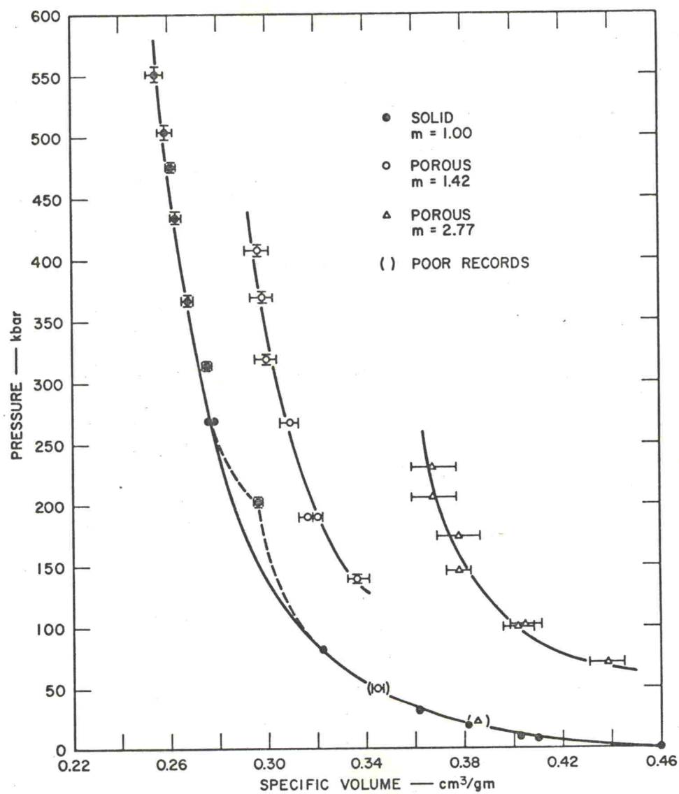
FIG. 6 TEFLON HUGONIOT DATA
